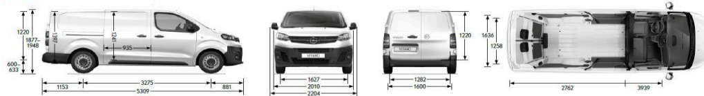
Vivaro Cargo L Alle Maße in mm
